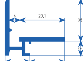
G5 26 x 27 mm maten tekening mm
